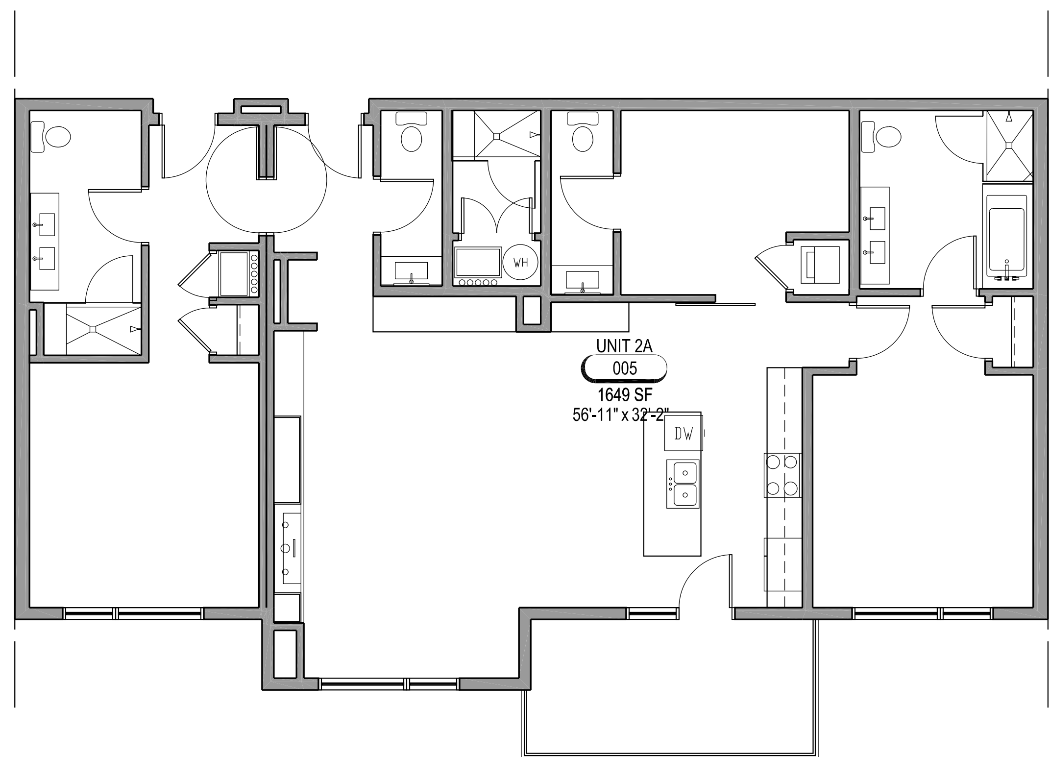
A1 UNIT TYPE 2A A401 SCALE: 3/16" = 1'-0"
